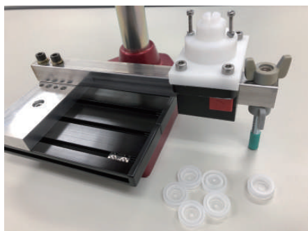
中栓セット前
